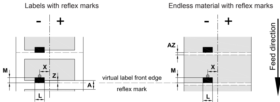
Fig. 15 Reflex mark dimensions
