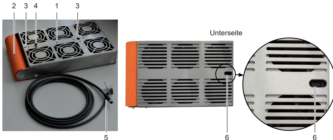
Roboter Kombistempel - Komponenten
