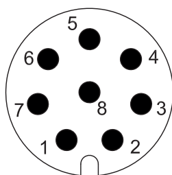
Belegung Flanschstecker
