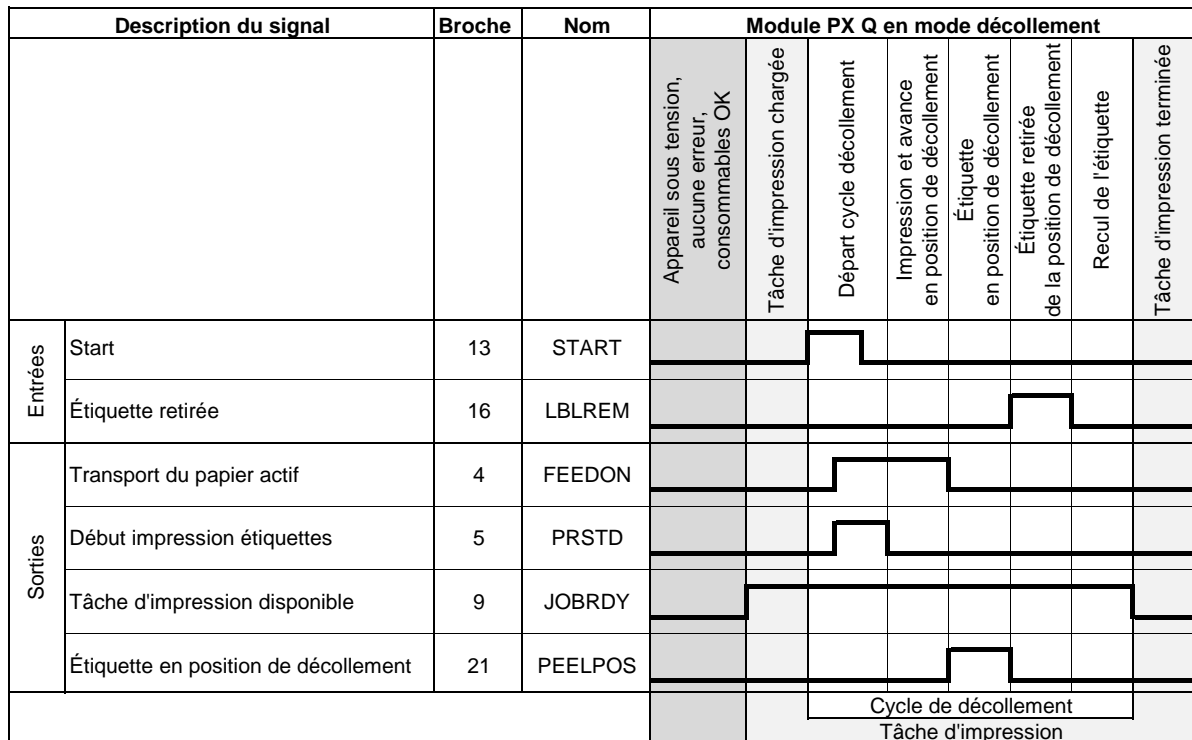
Figure 7 Chronogramme PX Q avec I/O 24V25-4 en mode décollement
