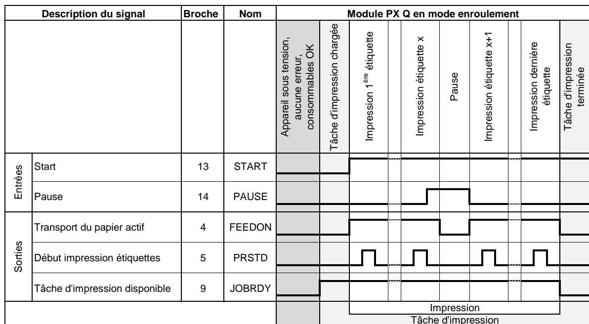
Figure 8 Chronogramme PX Q avec I/O 24V25-4 en mode enroulement
