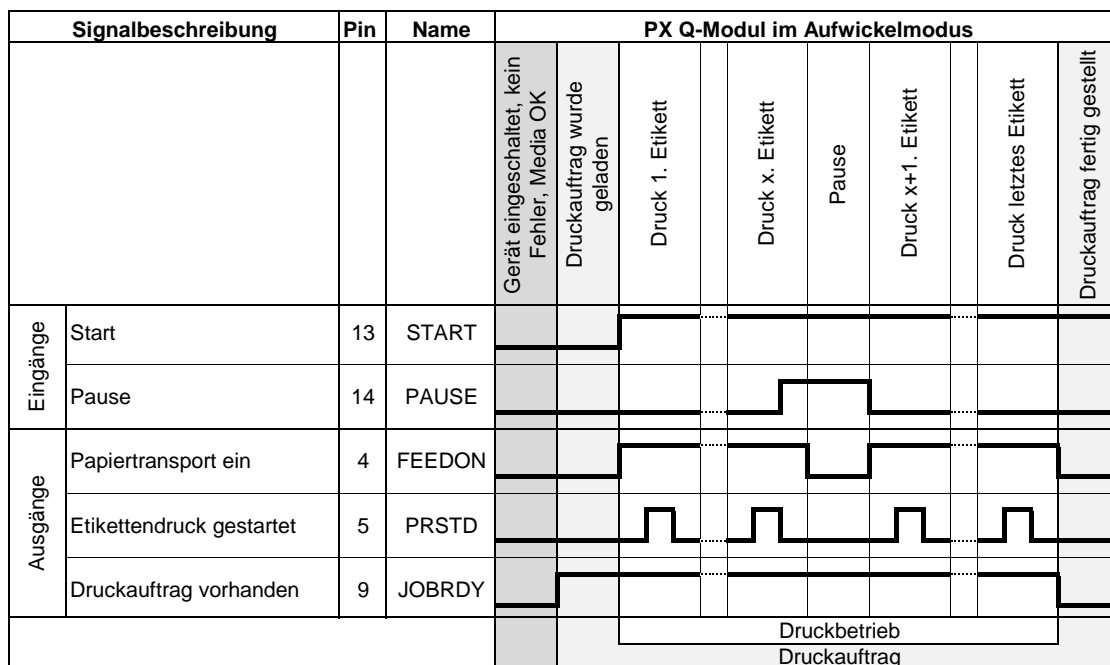
Bild 8 Signaldiagramm PX Q mit I/O 24V25-4 im Aufwickelmodus
