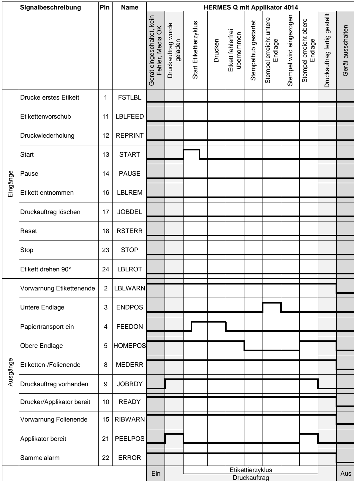
Bild 6 Signaldiagramm HERMES Q mit I/O 24V25-4 und Applikator 4014 im Modus "Drucken/Applizieren"
