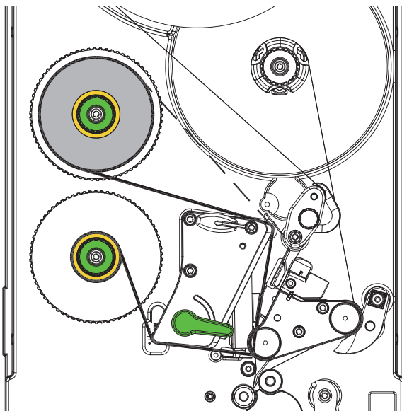
Figure 11 Passage du ruban transfert
