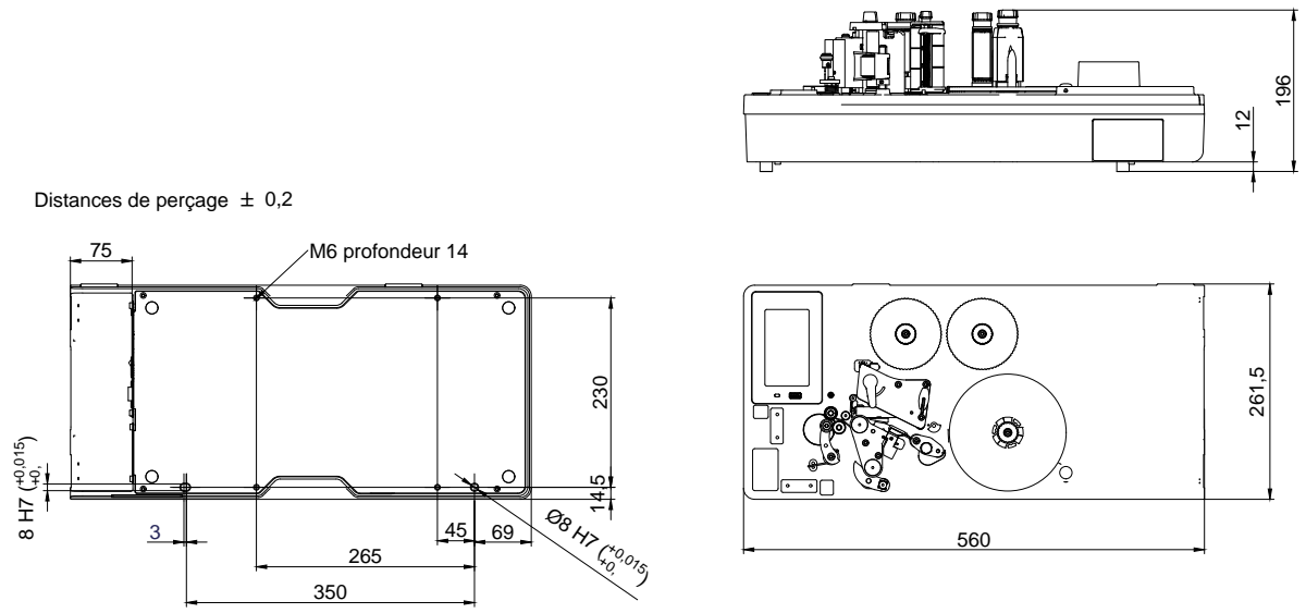
Figure 19 Dimensions d'intégration
