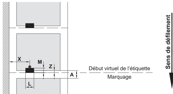
Figure 24 Dimensions des marques au dos
