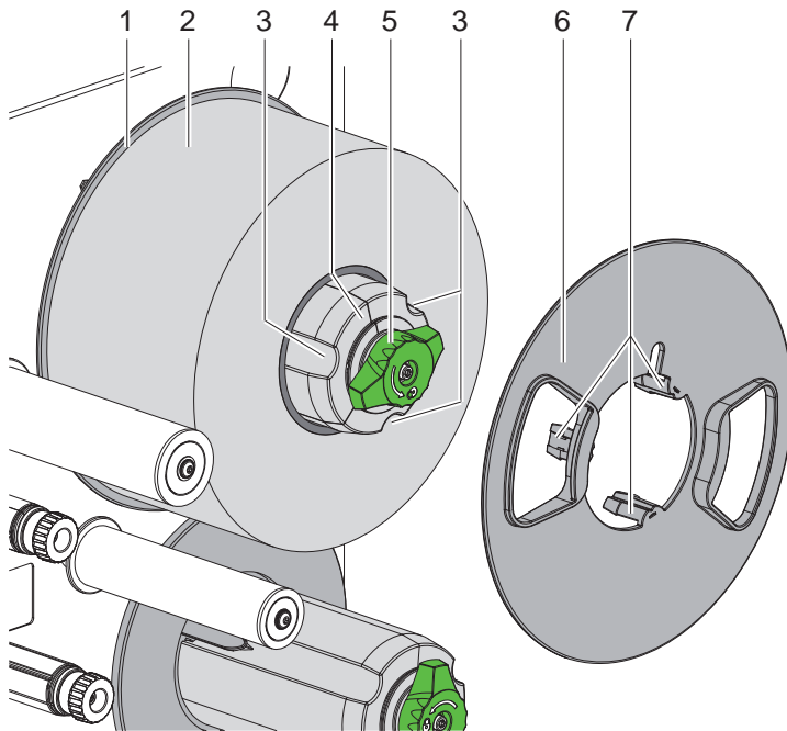
Figure 11 Insertion du rouleau d'étiquettes
