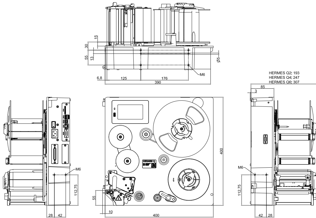
Figure 27 Dimensions d'intégration HERMES Q-2
