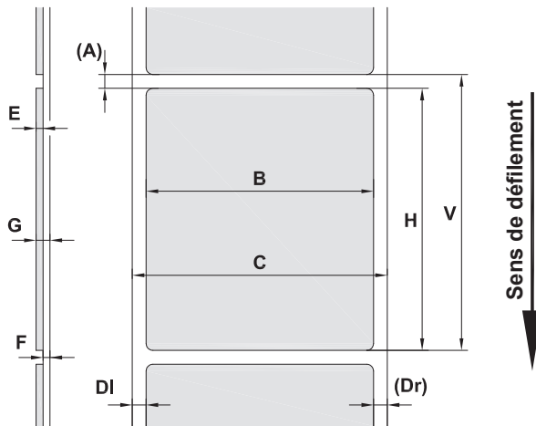
Figure 22 Dimensions des étiquettes
