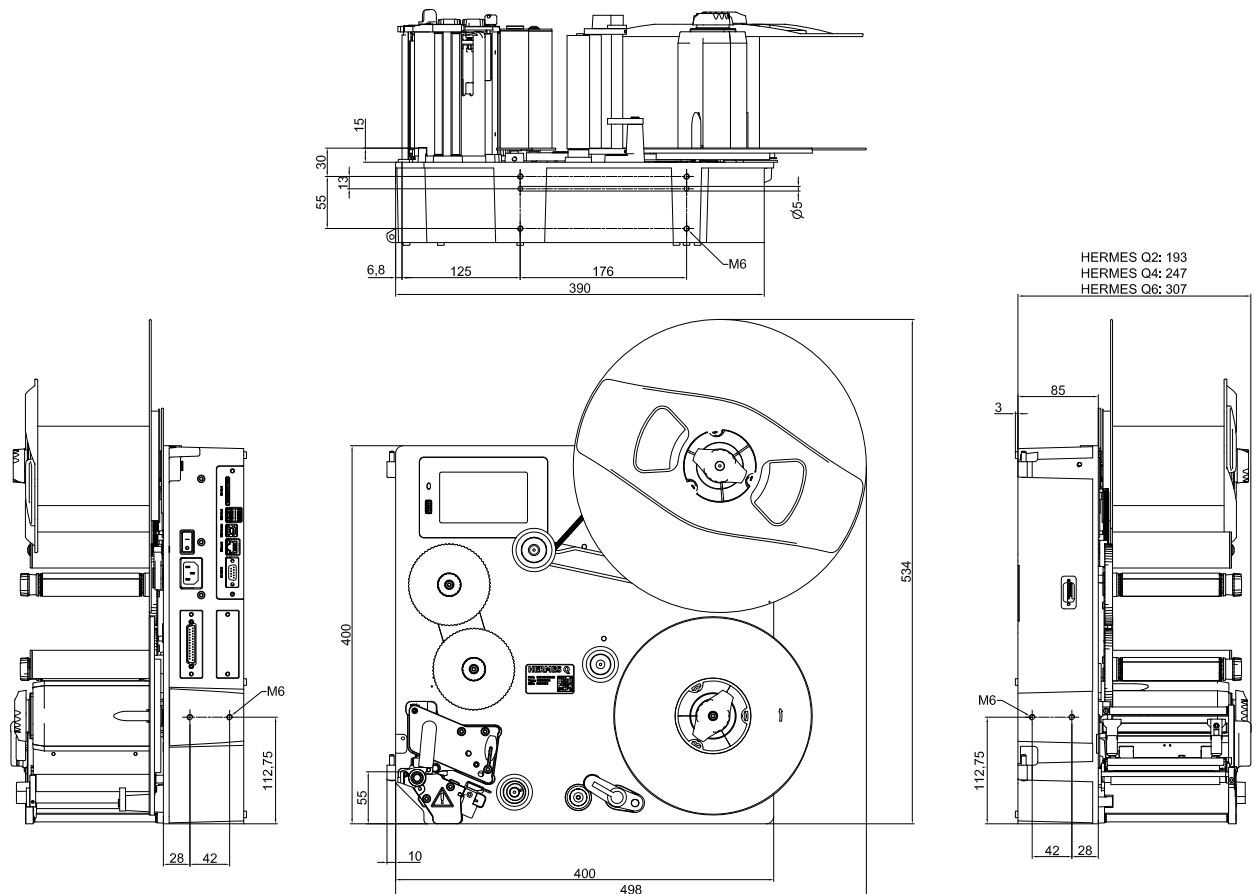
Figure 28 Dimensions d'intégration HERMES Q-3
