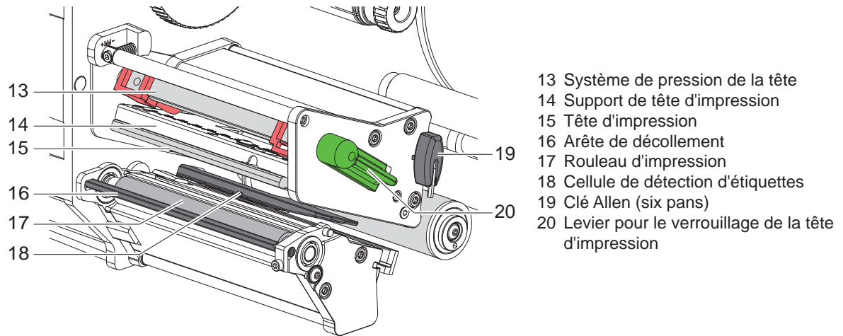
Figure 4 Mécanisme d'impression
