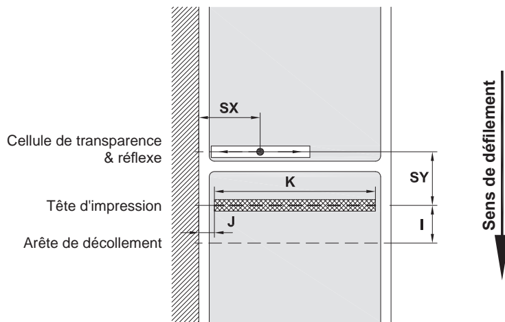
Figure 23 Dimensions de l'appareil
