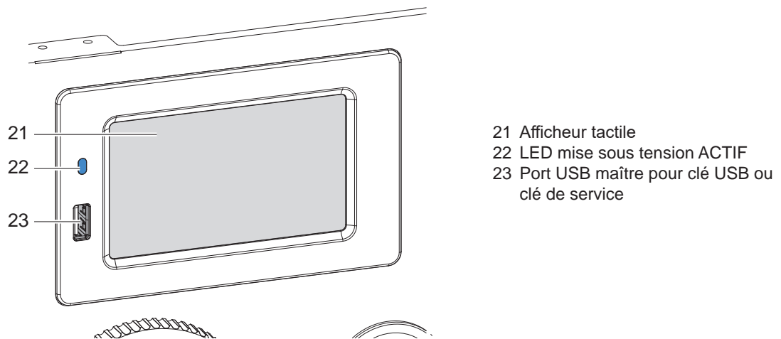
Figure 5 Panneau de commande
