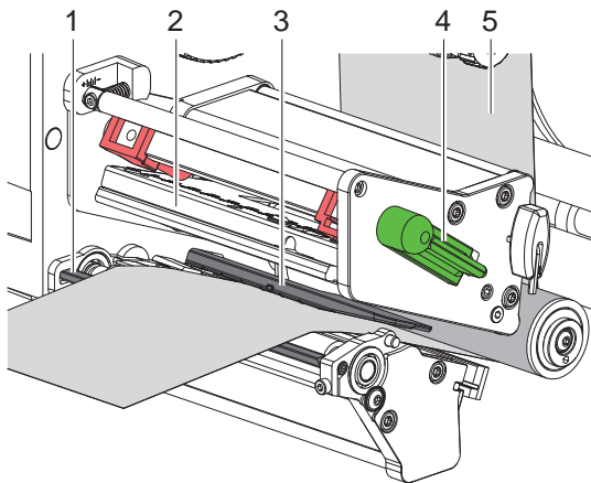
Figure 12 Insertion des étiquettes dans le mécanisme d'impression
