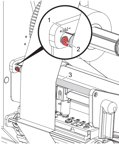
Figure 20 Réglage du défilement du ruban transfert
