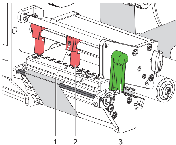
Figure 16 Réglage du système de pression de la tête d'impression
