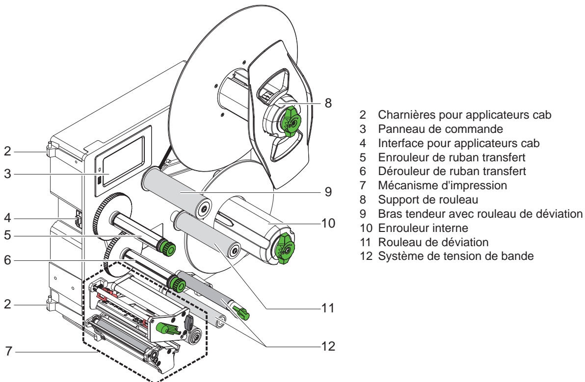
Figure 3 Vue d'ensemble HERMES Q-3
