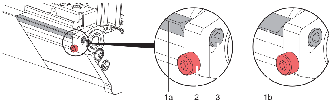
Figure 17 Réglage de l'arête de décollement
