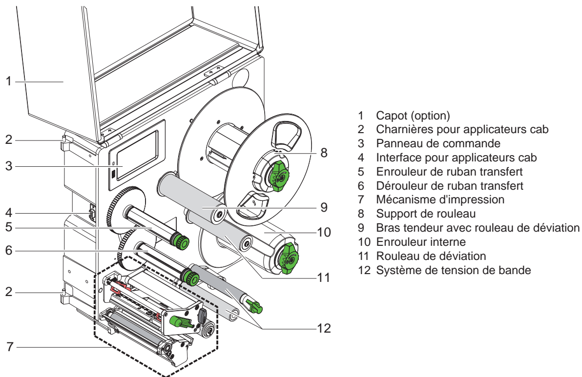
Figure 2 Vue d'ensemble HERMES Q-2
