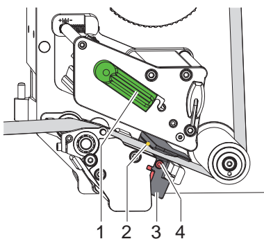
Figure 14 Réglage de la cellule de détection d'étiquettes
