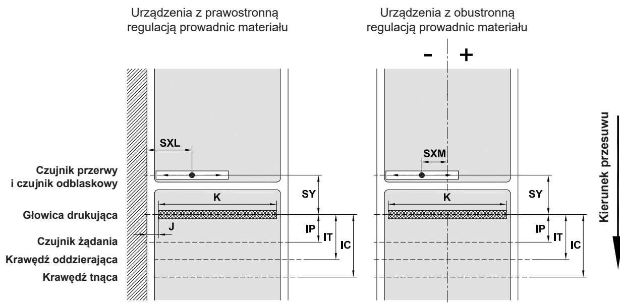
Ilustracja 31 Wymiary urządzenia
