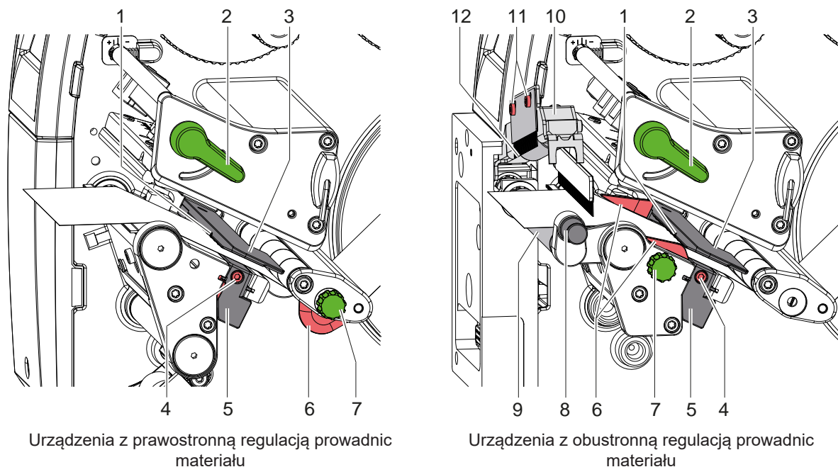
Ilustracja 16 Wkładanie etykiet do głowicy drukującej
