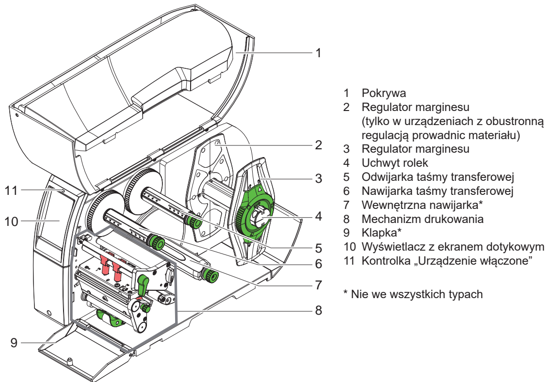
Ilustracja 1 Budowa
