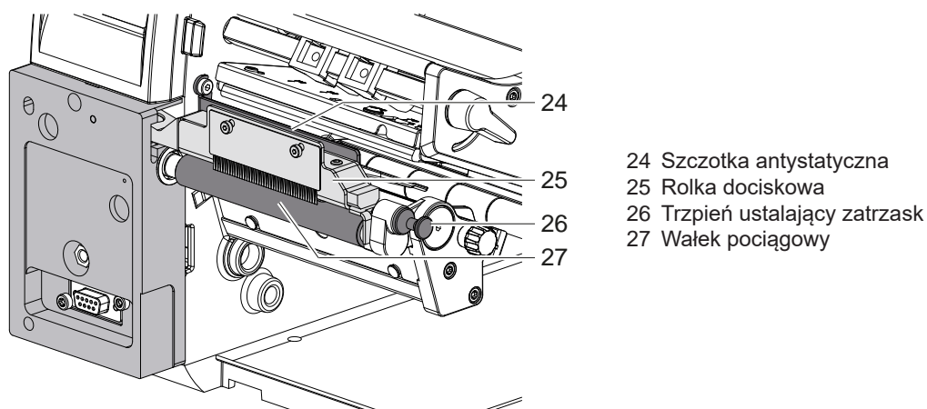
Ilustracja 6 Separator w SQUIX MT
