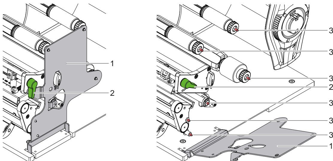
Ilustracja 14 Wspornik kątowy SQUIX 8.3
