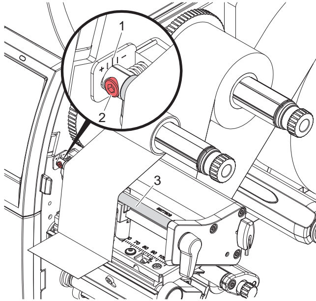
Ilustracja 27 Ustawianie przebiegu taśmy transferowej
