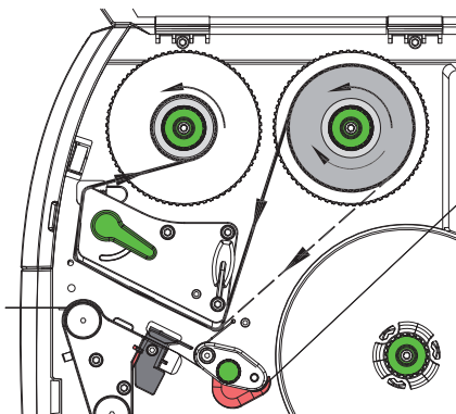
Ilustracja 26 Przebieg taśmy transferowej
