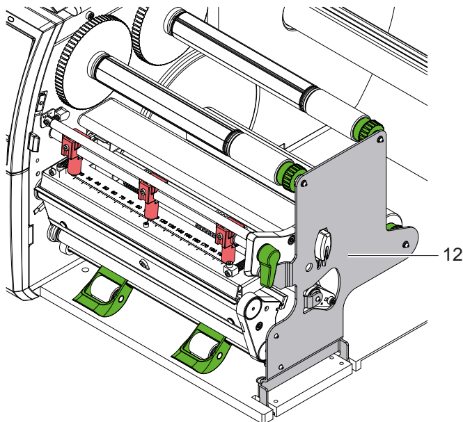
Ilustracja 2 Wspornik SQUIX 8.3
