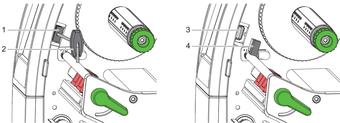
Ilustracja 8 Wkładanie karty wtykowej Wi-Fi
