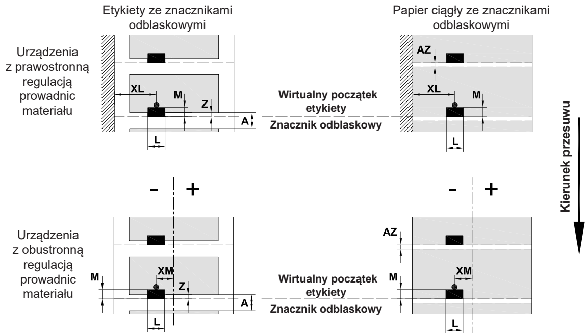
Ilustracja 32 Wymiary znaczników odblaskowych
