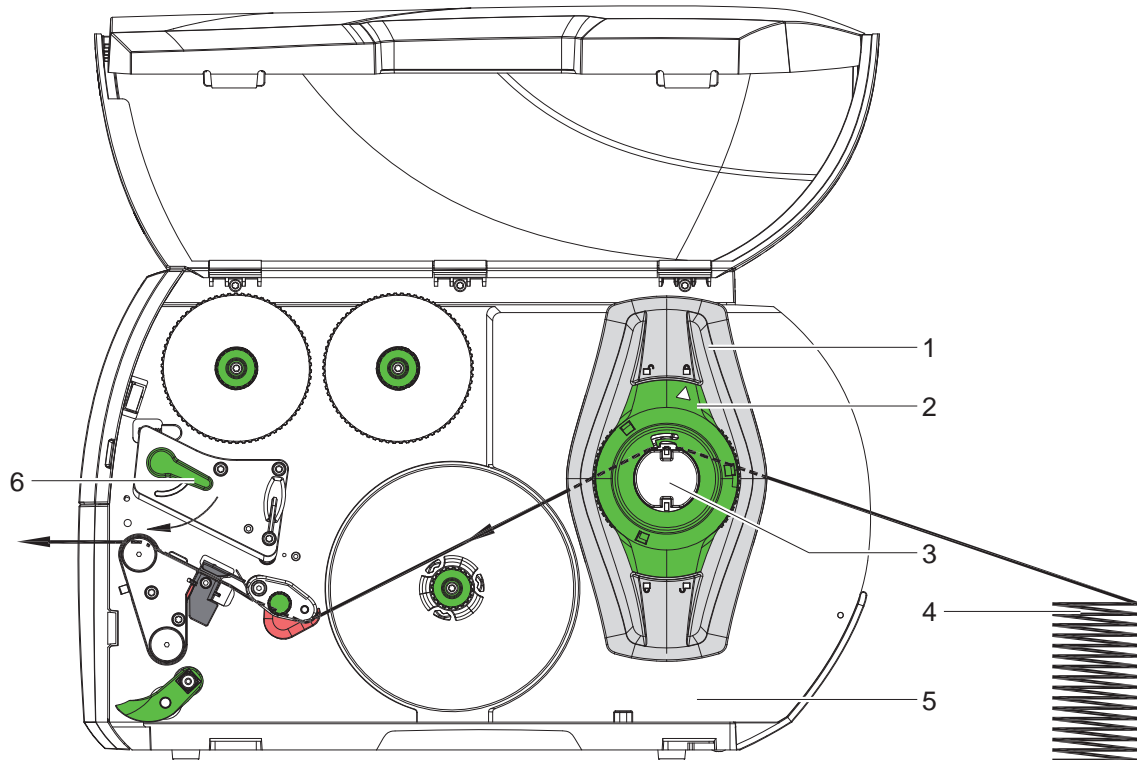
Ilustracja 21 Przebieg papieru z etykietami leporello
