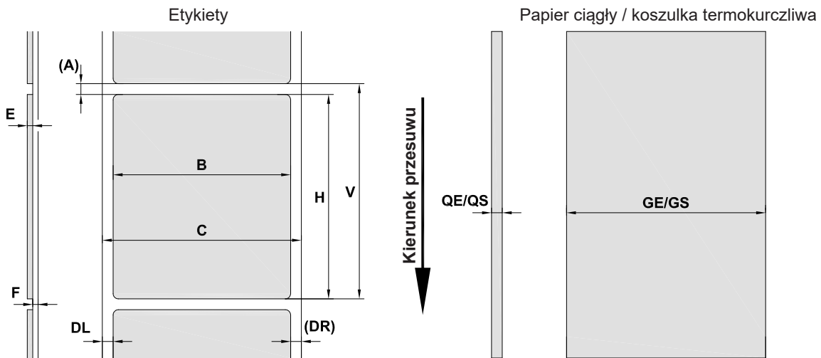
Ilustracja 30 Wymiary etykiet / papieru ciągłego
