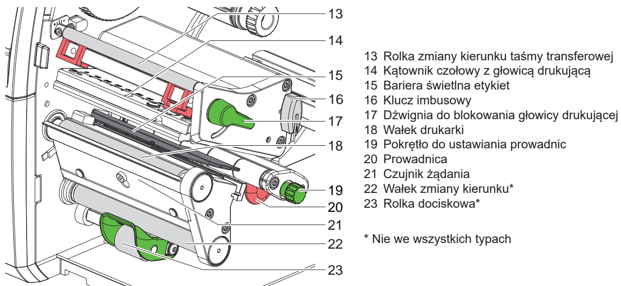
Ilustracja 3 Mechanizm drukowania — urządzenia z prawostronną regulacją prowadnic materiału (z wyjątkiem SQUIX 8.3)
