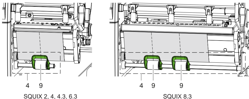
Ilustracja 20 Wyrównanie rolek dociskowych
