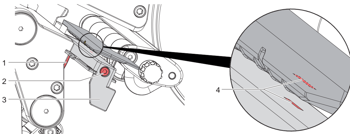
Ilustracja 28 Czyszczenie bariery świetlnej etykiet
