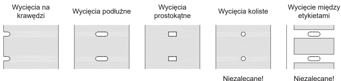
Ilustracja 34 Przykładowe wycięcia
