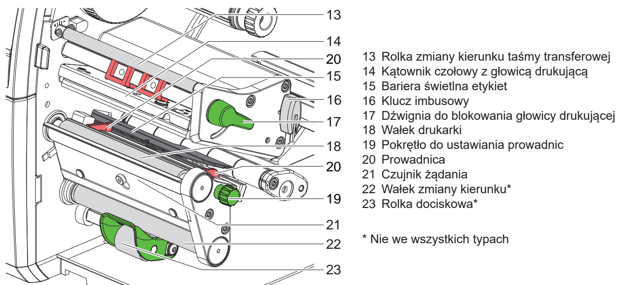
Ilustracja 5 Mechanizm drukowania — urządzenia z obustronną regulacją przewodnic materiału
