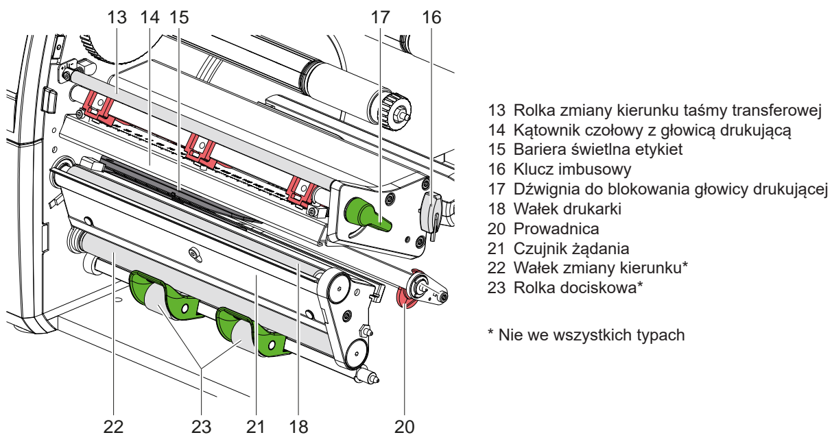
Ilustracja 4 Mechanizm drukowania SQUIX 8.3
