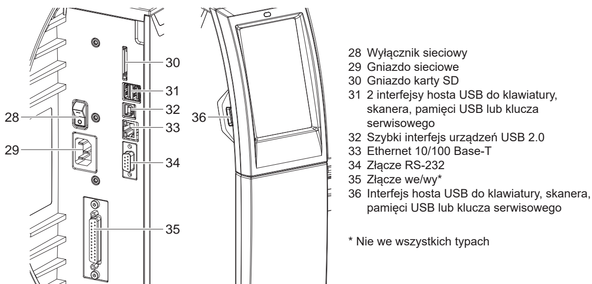
Ilustracja 7 Przyłącza
