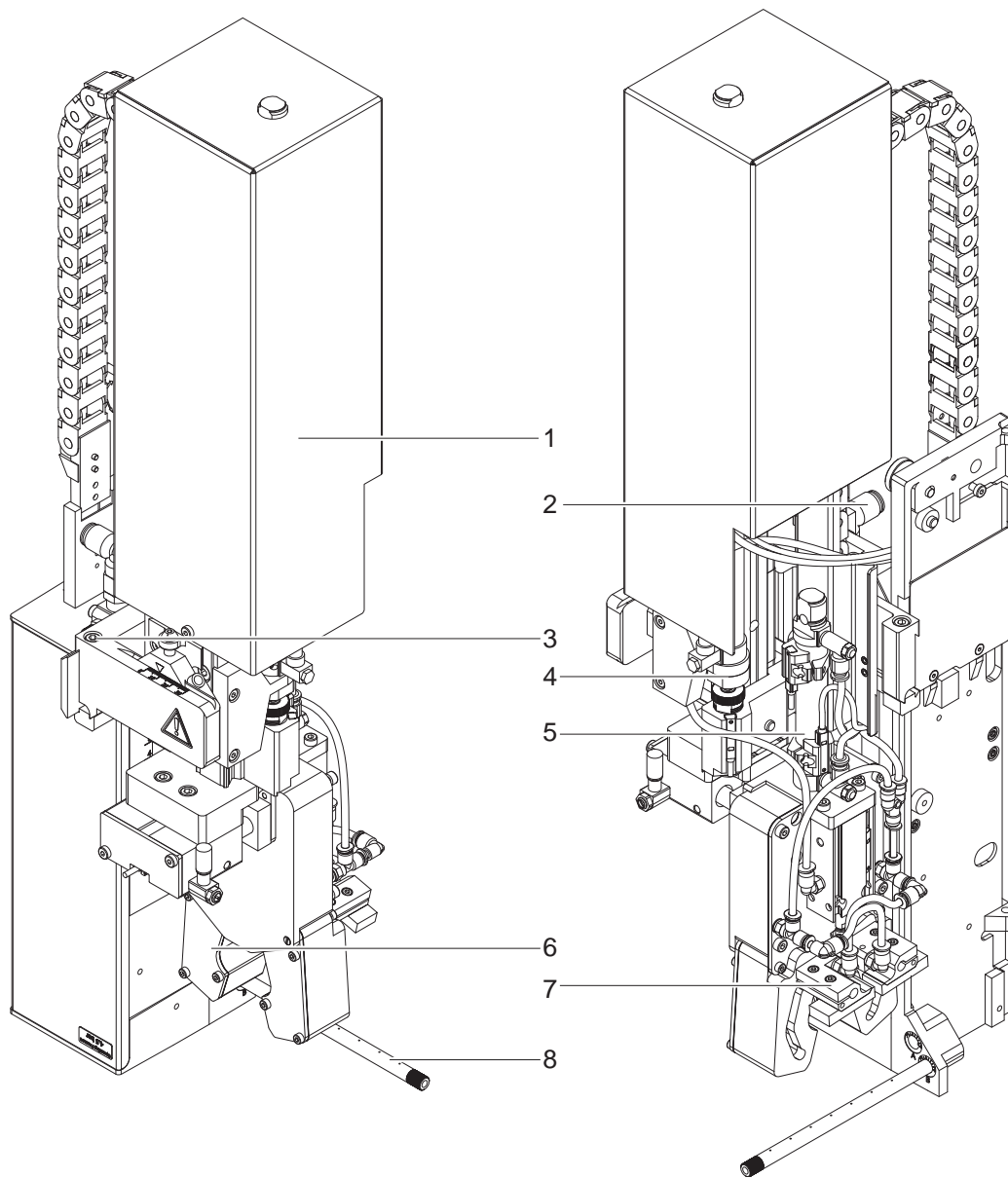
Bild 3 Geräteübersicht
