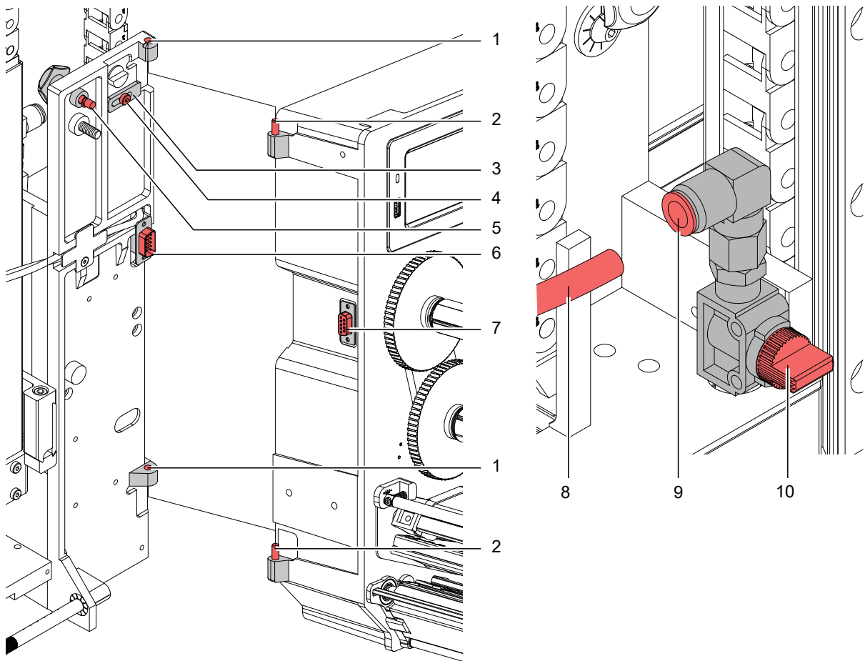
Figure 4 Montage et démontage de l'applicateur
