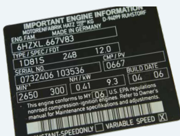
Placas de características de aluminio
